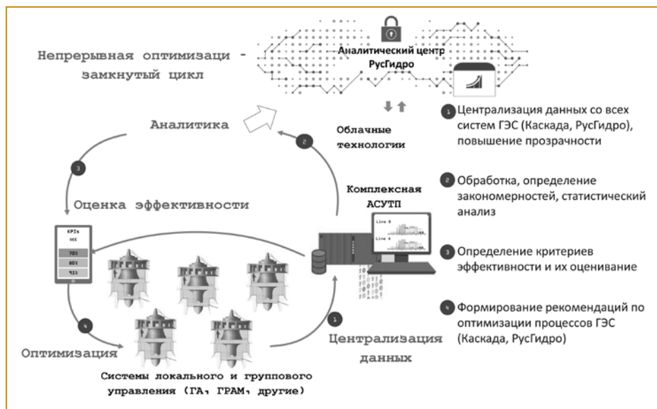
Рис. 2. Схема оптимизации работы ГЭС
