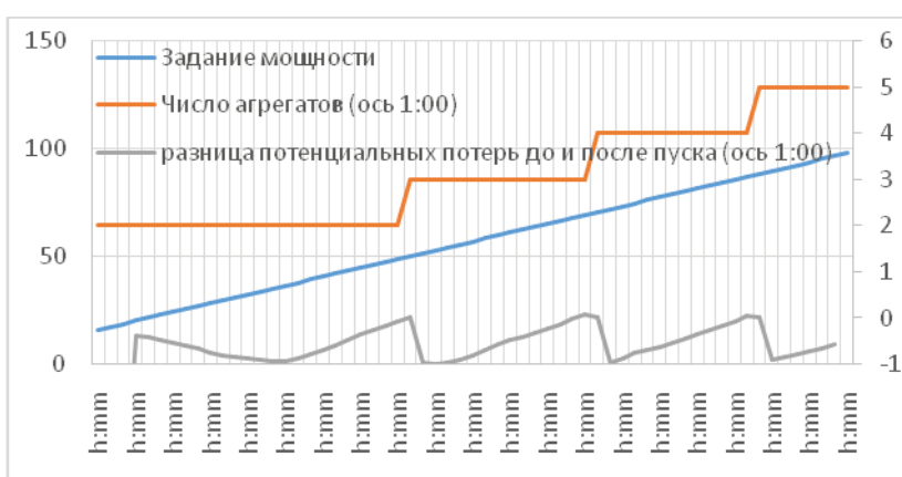
Рис.3 Оптимальное изменение состава агрегатов при росте загрузки
