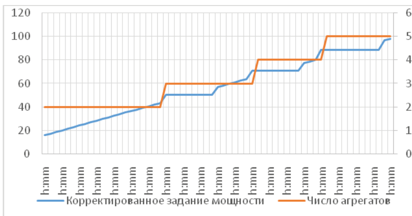
Рис.4 Оптимальное изменение состава агрегатов при росте загрузки с корректированным заданием ГЭС
